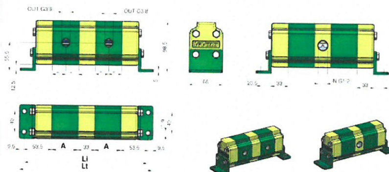
FLOW DIVIDERS | ΧΩΡΙΣ ΒΑΛΒΙΔΑ GROUP 1
