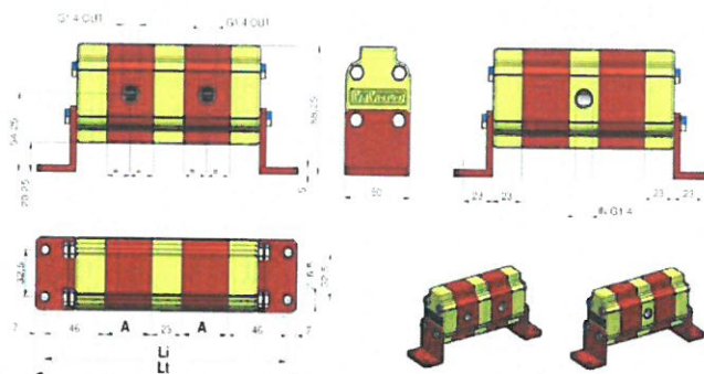
FLOW DIVIDERS | ΧΩΡΙΣ ΒΑΛΒΙΔΑ GROUP 0
